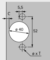
complètement en applique (base B 18 mm)
