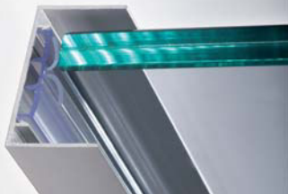
3 Raamprofiel Robustus
