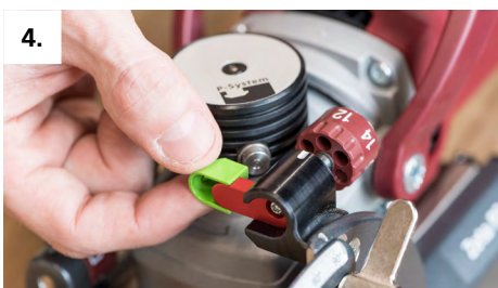
4. Monter l'outil de réglage de profondeur P-System de 4 mm (profondeur de fraisage effective : 8 mm)
